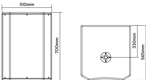
Pro-515S尺寸图
