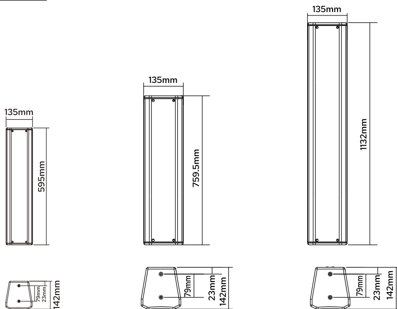
Pro-403尺寸图
